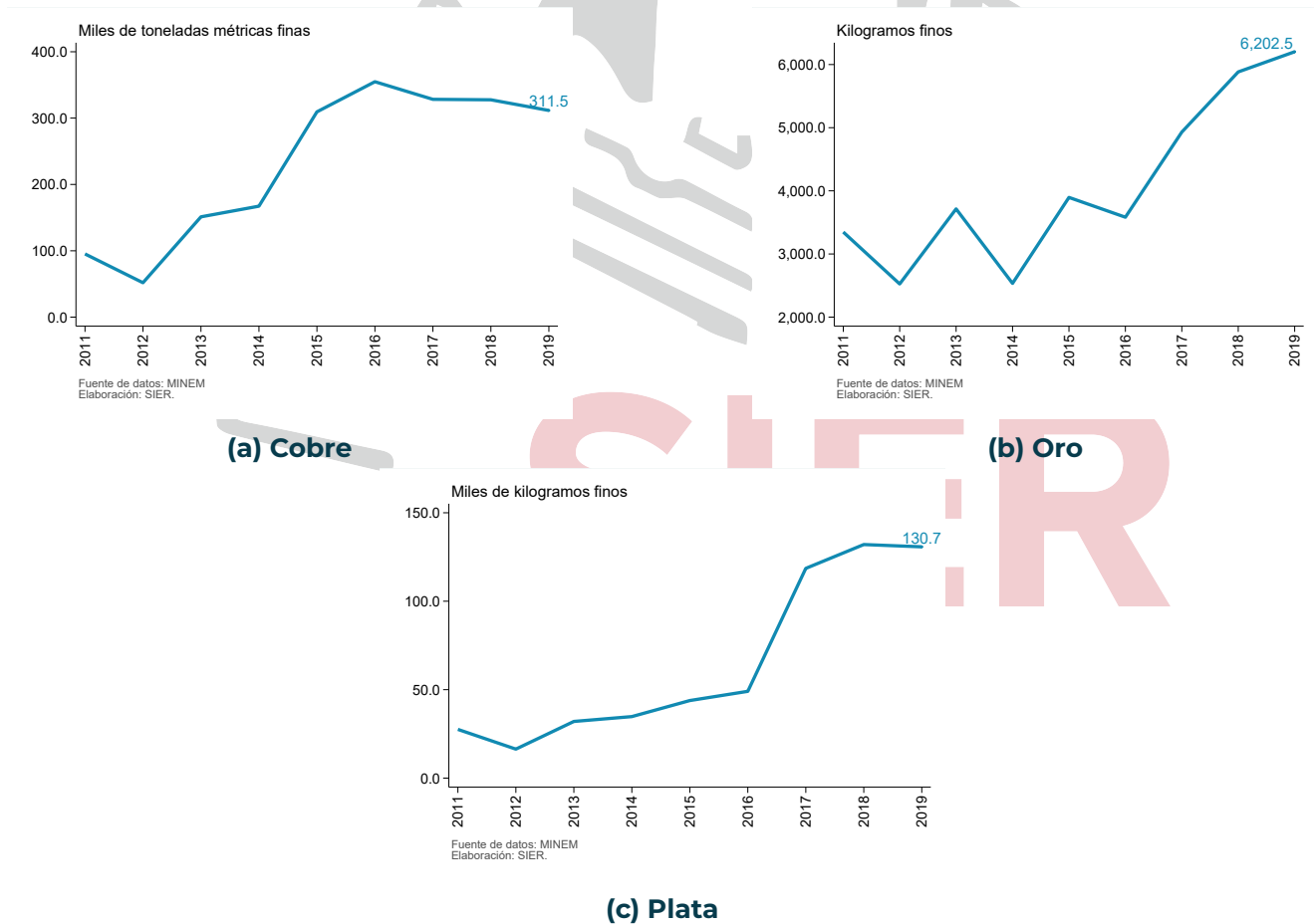
Figura 7.1: Producción Minera Metálica en Cusco al 2019
